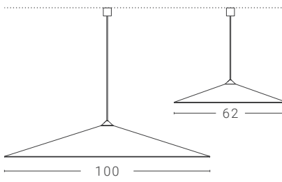
Jeena sospensione - Versione C Jeena suspension - Version C
