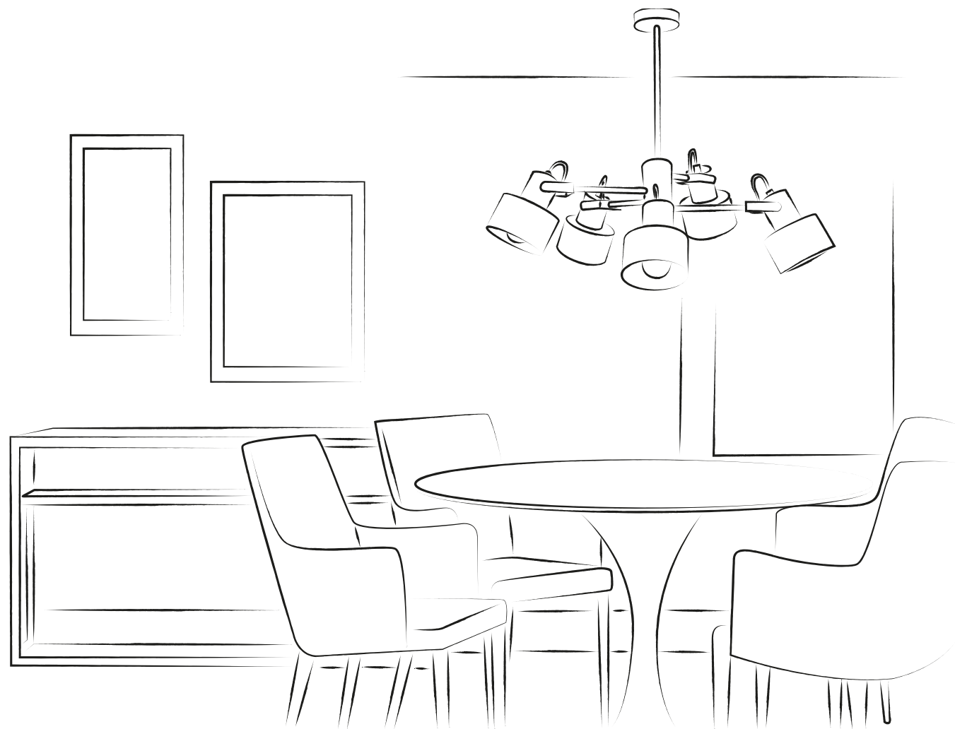
1 METRO 5 31580 czarny / black 31581 biały / white 5 × E27 160 –53 /53 Δ 7,5 Ø 12
