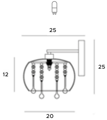
W0076-01D 1x40W G9 230V chrom chrome szkło lustrzane, metal mirror glass, metal
