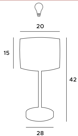
T0010 1x60W E27 230V chrom, biały abażur chrome, white shade metal, tkanina metal, fabric
